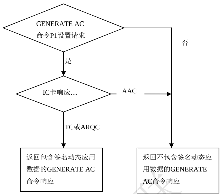
图4 CDA 处理流程一卡片 GENERATE AC 命令处理
